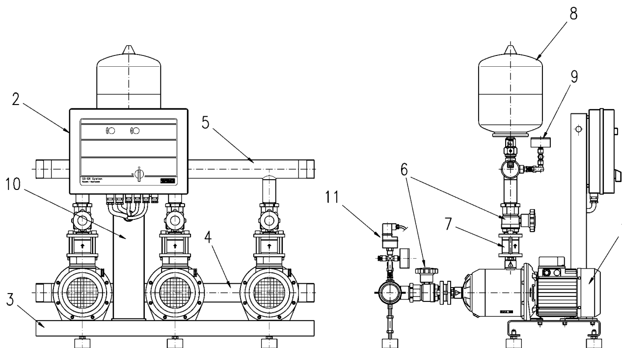
Рис. 1а. Установка DEA с насосами МНІ и устройством регулирования ER
