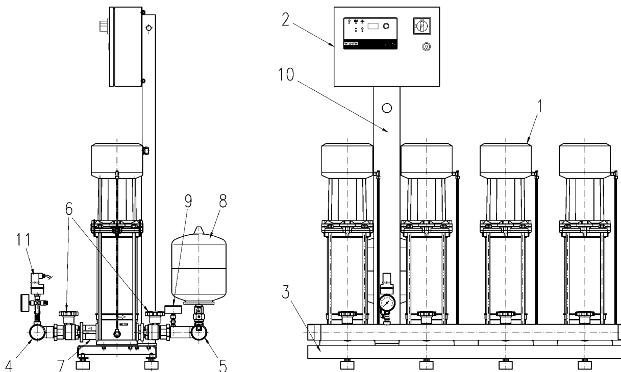
Рис. 1б. Установка DEA с насосами MVISE и устройством регулирования VR
