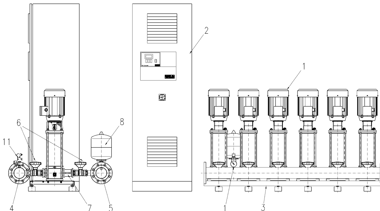
Рис. 1с. Установка DEE с насосами MVI и устройством регулирования CR в отдельно стоящем шкафу
