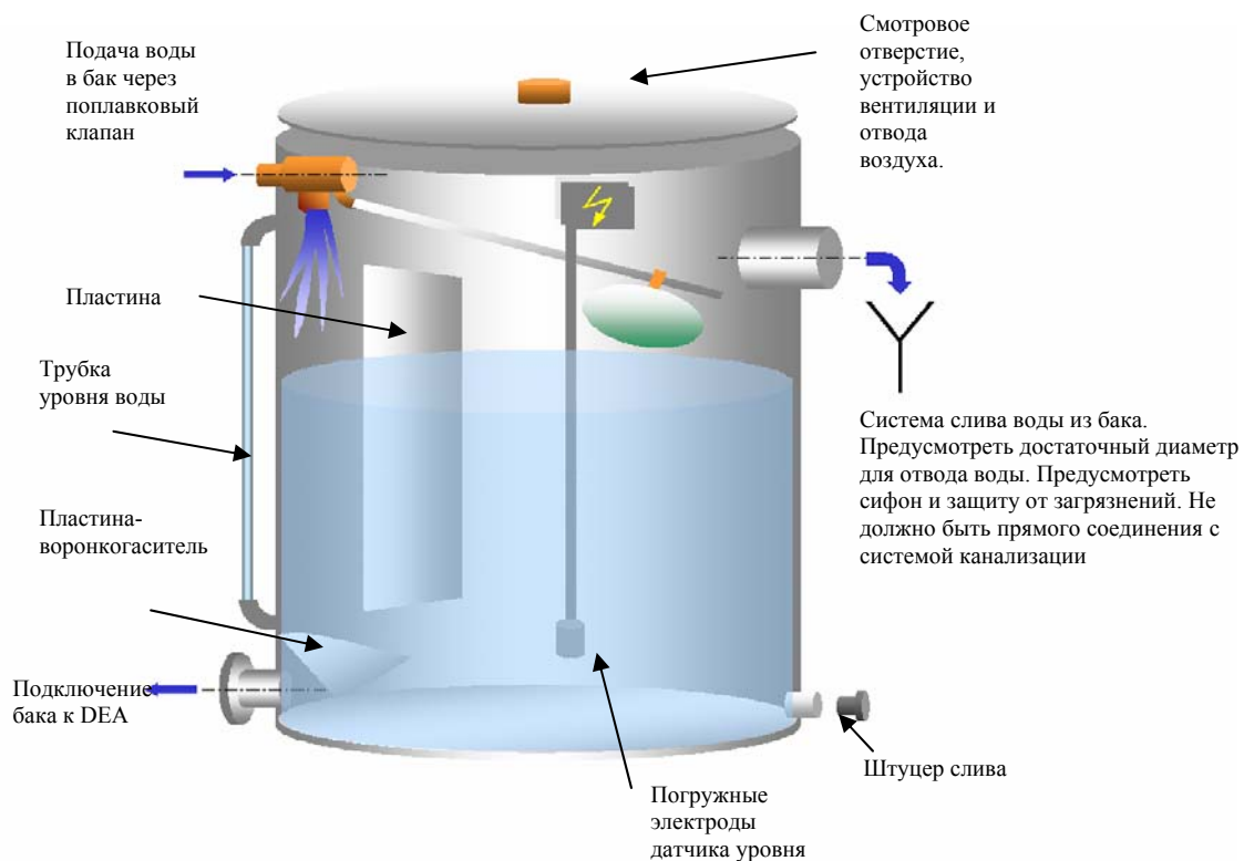
Рис. 9. Накопительный бак открытого типа
