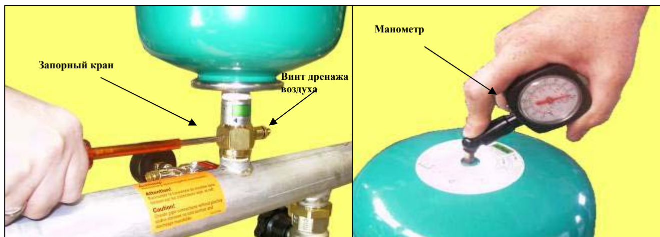
Рис. 2б. Обслуживание мембранного бака и проверка давления его наддува
