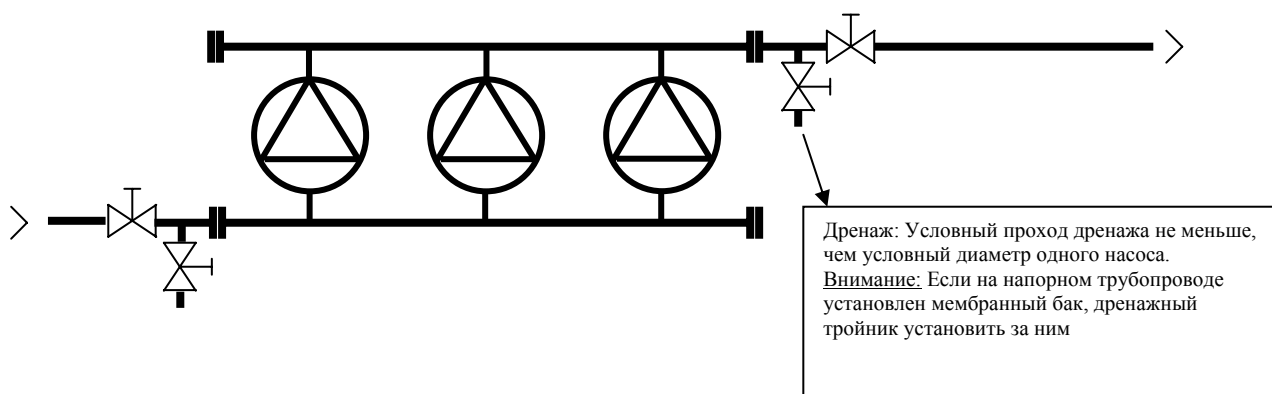
Рис. 10. Схема промывки DEA
