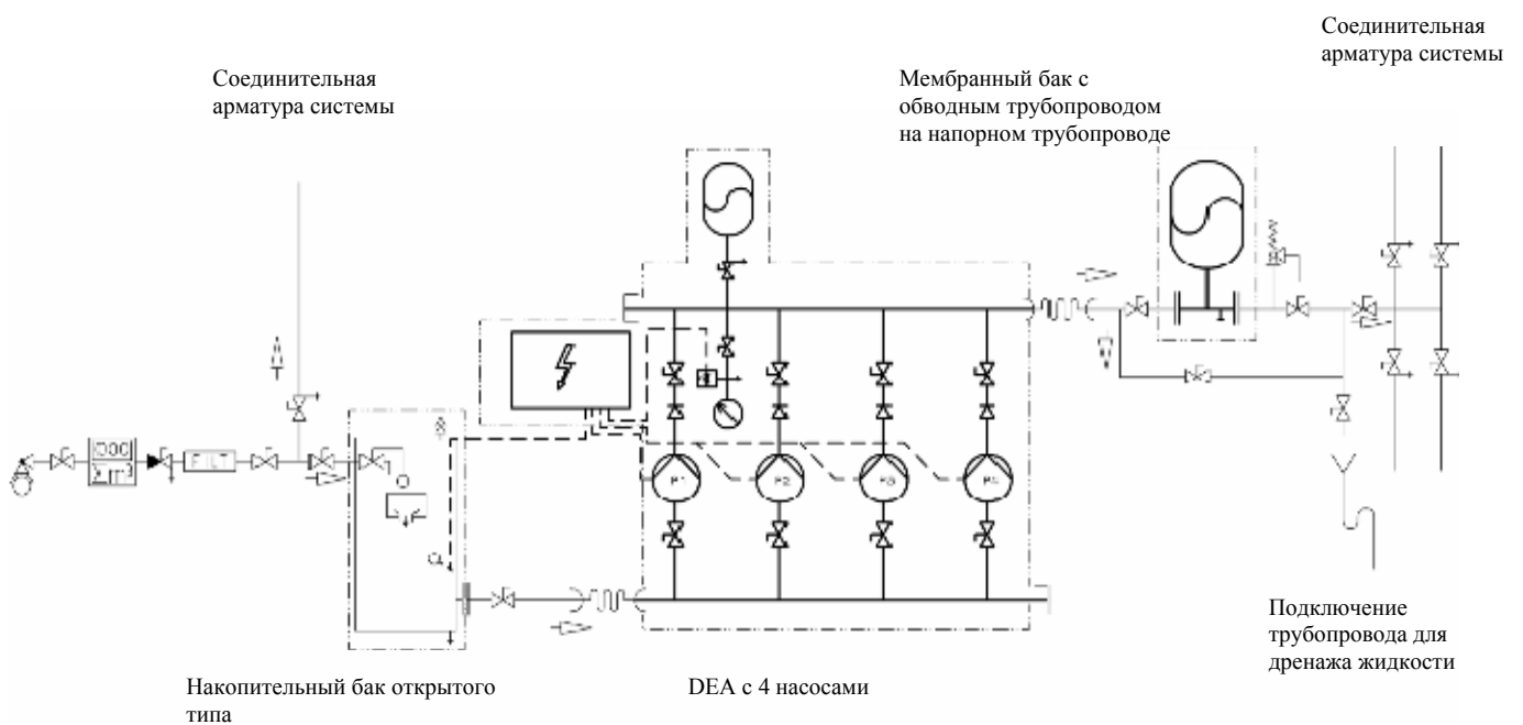
Рис. 6. Подключение DEA к водопроводной сети через накопительный бак открытого типа
